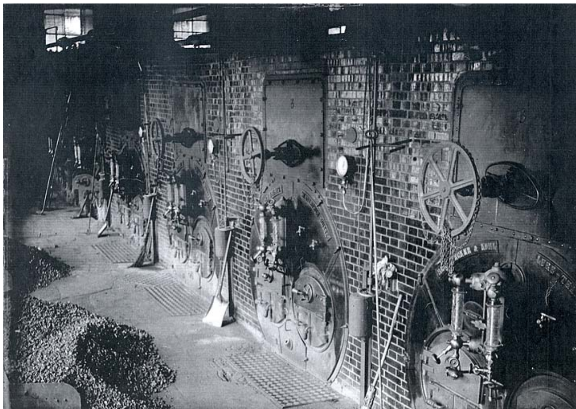
Chaudières à charbon Scheidecker et Kohl.
