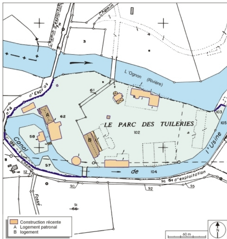
Plan-masse et de situation. Extrait du plan cadastral numérisé, 2006, section ZB, 1:1200.
