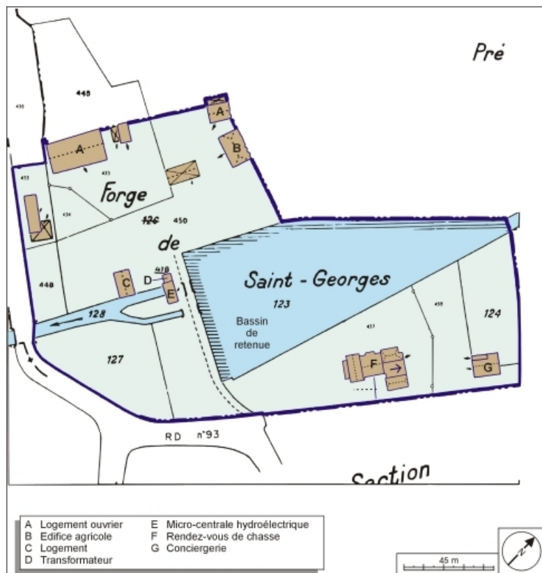
Plan-masse et de situation. Extrait du plan cadastral numérisé, 2005, section A, 1:1250 réduit à 1:1500. 70, Athesans-Étroitefontaine, lieudit : Saint-Georges
