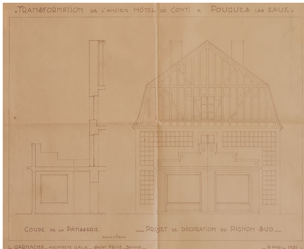
Projet de construction d'une pâtisserie, élévation et coupe (1931).
