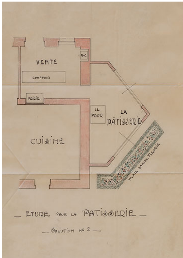
Projet de construction d'une pâtisserie, plan (1931).
