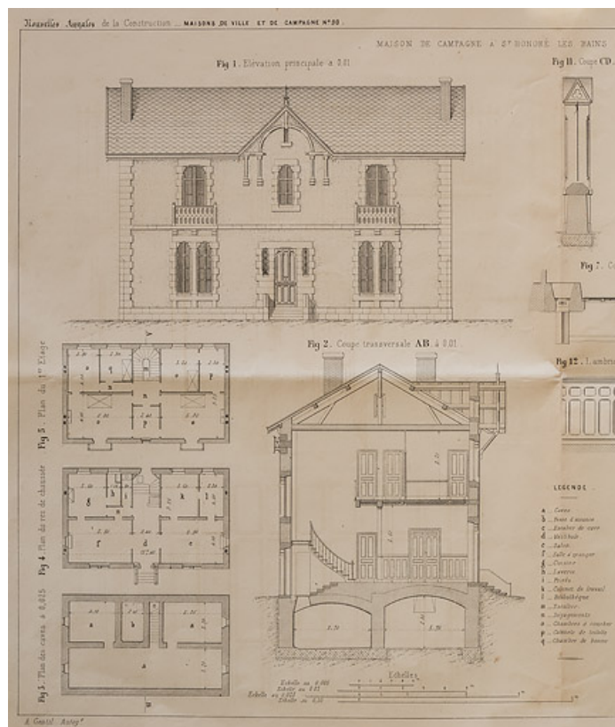
Élévation principale, coupe transversale, plans des caves, du rez-de-chaussée et de l'étage. 58, Saint-Honoré-les-Bains, 4 avenue de Rémyilly
