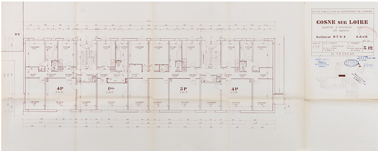
Opération de 226 logements : bâtiment B3, plan du rez-de-chaussée ; J. Louria, F. Sonnet, avril 1969. (Archives municipales Cosne-Cours-sur-Loire, 200 W 117 - PC 1015) 58, Cosne-Cours-sur-Loire avenue de la Paix
