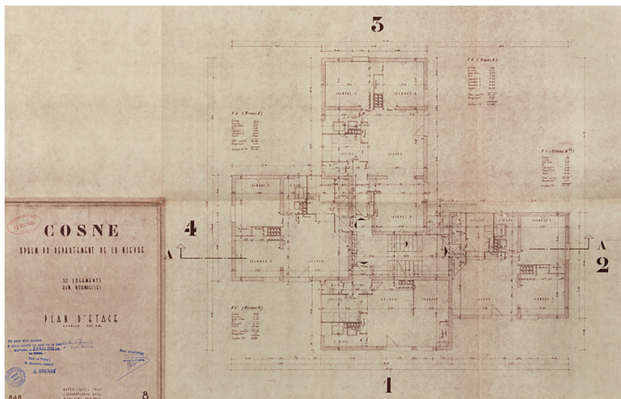
Opération de 32 logements, plan d'étage, L. Robert et M. Guillaume, avril 1955. (Archives municipales Cosne-Cours-sur-Loire, 200 W 16 - PC 722)
