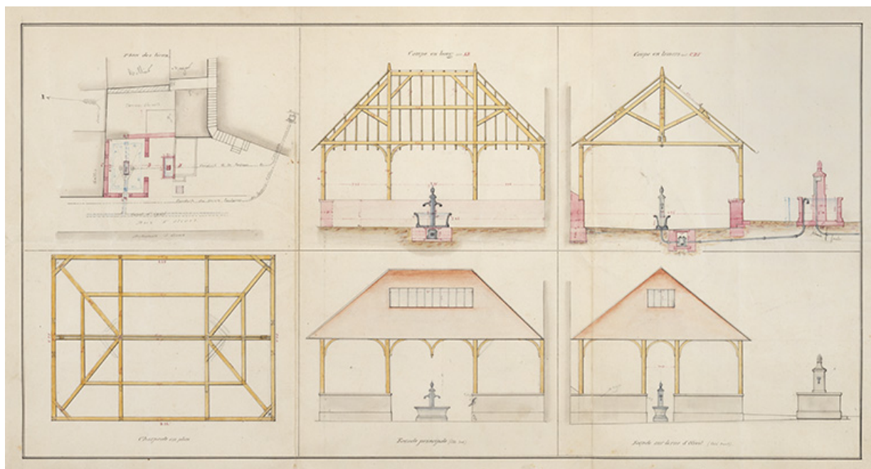
Lavoirs - Plans, coupes et élévations, 1879.
