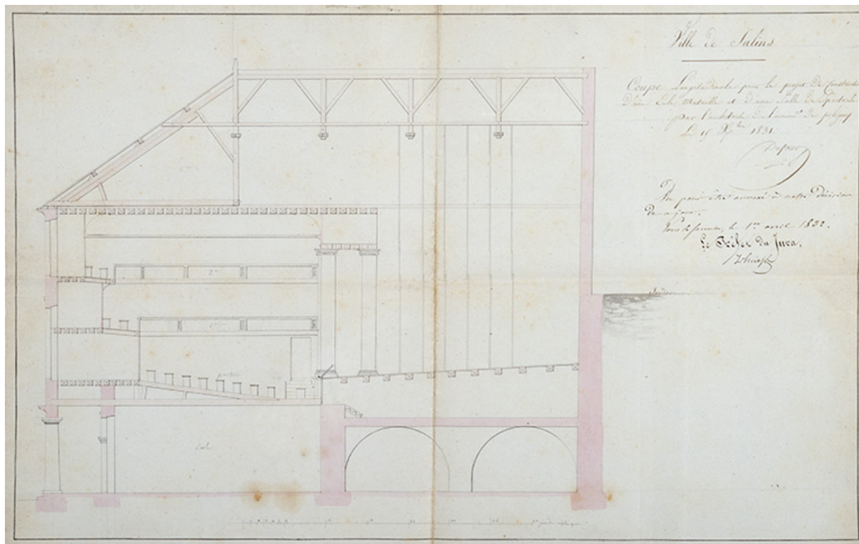
Coupe longitudinale pour le projet de construction d'une école mutuelle et d'une salle de spectacle, 1831. 39, Salins-les-Bains rue de la République
