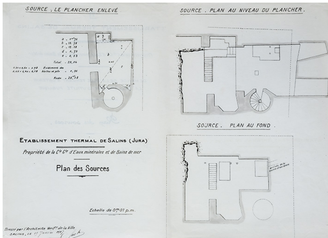
Plans du sous-sol du Grand Hôtel des Bains, figurant le puits à Muire (1917).
