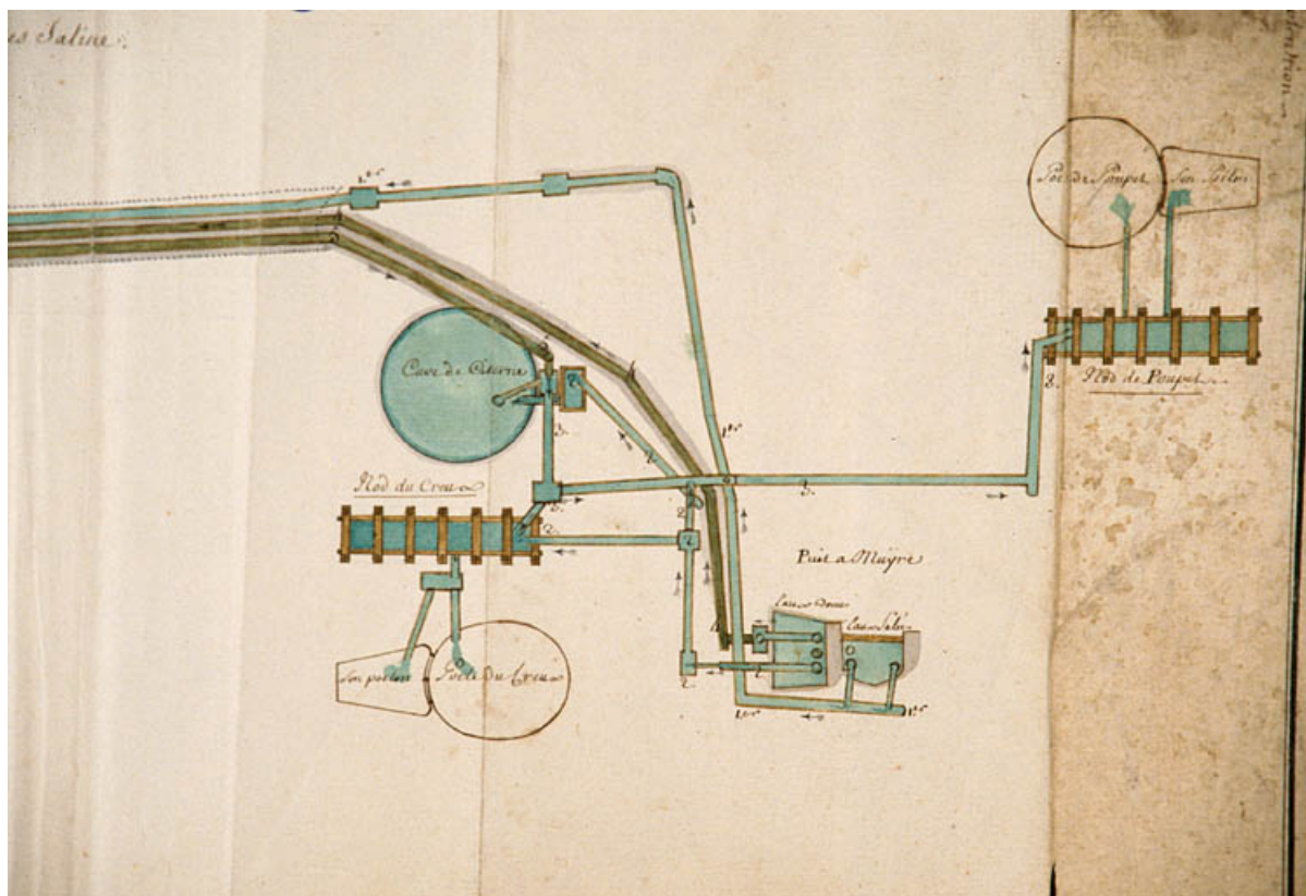
Plan des Différents Cours des Eaux salées et douces [... : détail du puits à muire et des bernes du Creux et du Poupet]. 39, Salins-les-Bains, 2 place des Alliés et de la Résistance
