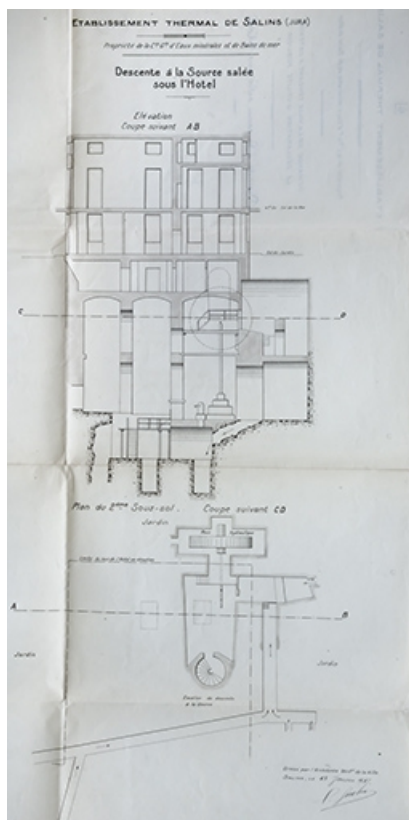
Coupes du sous-sol du Grand Hôtel des Bains, figurant le puits à Muire (1917).
