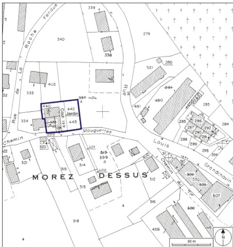
Plan-masse et de situation. Extrait du plan cadastral, 1980, section AI, échelle 1:1000. 39, Morez, 4 à 8 chemin des Mouguettes
