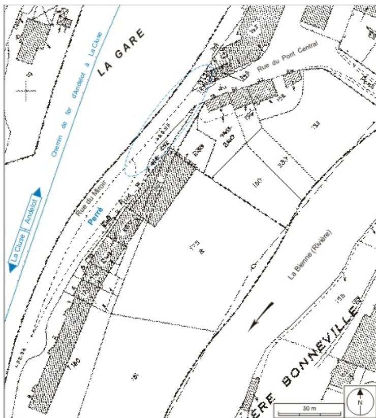
Plan-masse et de situation. Extrait du plan cadastral, 1980, section AH, échelle 1:1000. 39, Saint-Claude rue du Miroir
