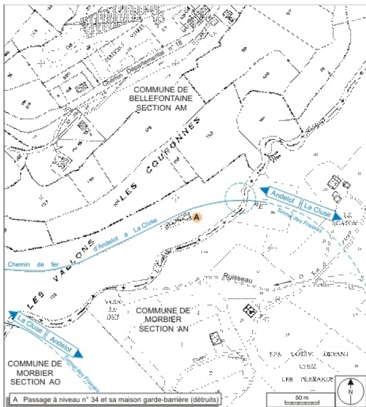
Plan-masse et de situation. Montage d'extraits du plan cadastral, Bellefontaine, 1983, section AM (1:2000), et Morbier, 2006, section AN, échelle 1:3000.
