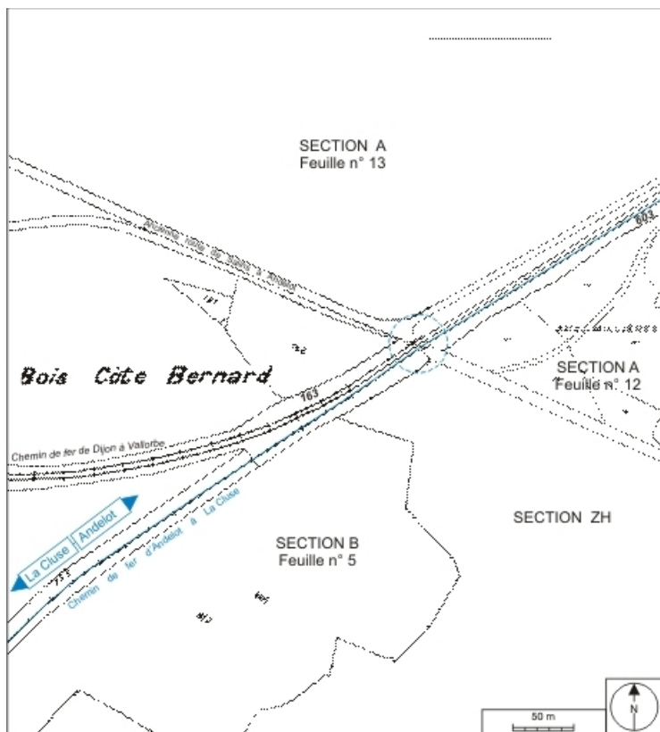
Plan-masse et de situation. Montage d'extraits du plan cadastral, 1995, sections A (12e feuille, 1:1250) et B (5e feuille, 1:2500), réduit à 1:3000.
