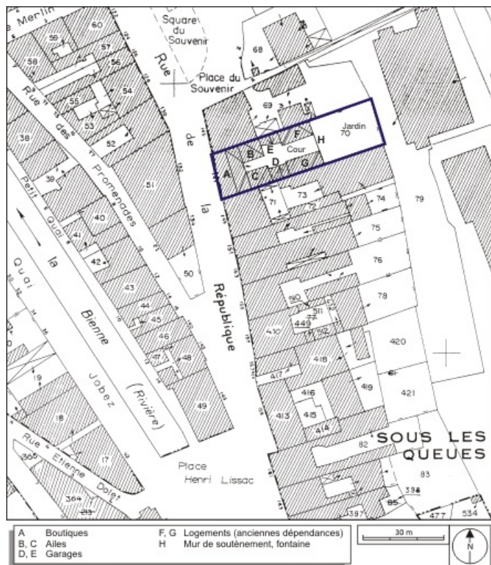
Plan-masse et de situation. Extrait du plan cadastral, 1980, section AI, échelle 1:1000. 39, Morez, 147 rue de la République
