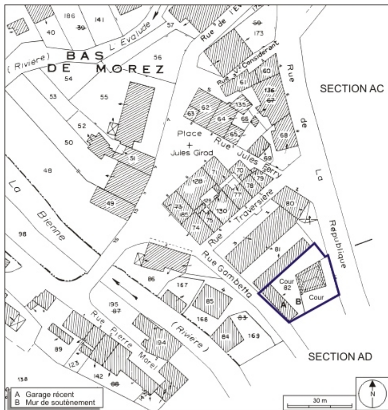
Plan-masse et de situation. Extrait du plan cadastral, 1980, section AB, échelle 1:1000. 39, Morez, 14 rue de la République
