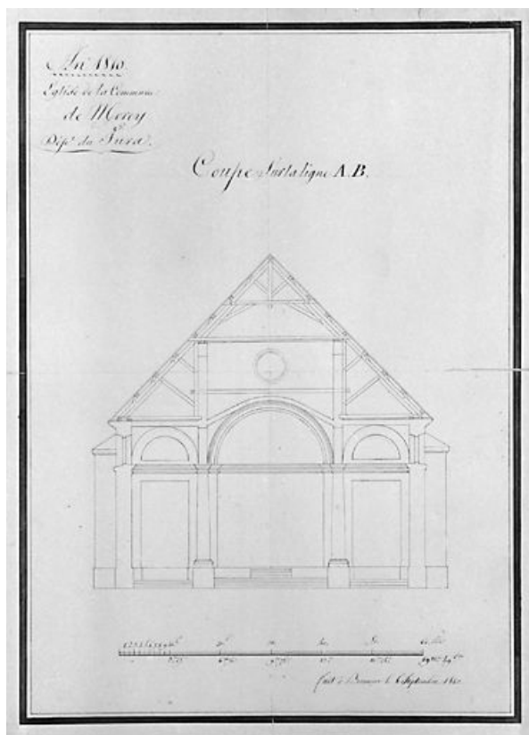
An 1810. Eglise de la commune de Morez. Coupe sur la ligne A.B.
