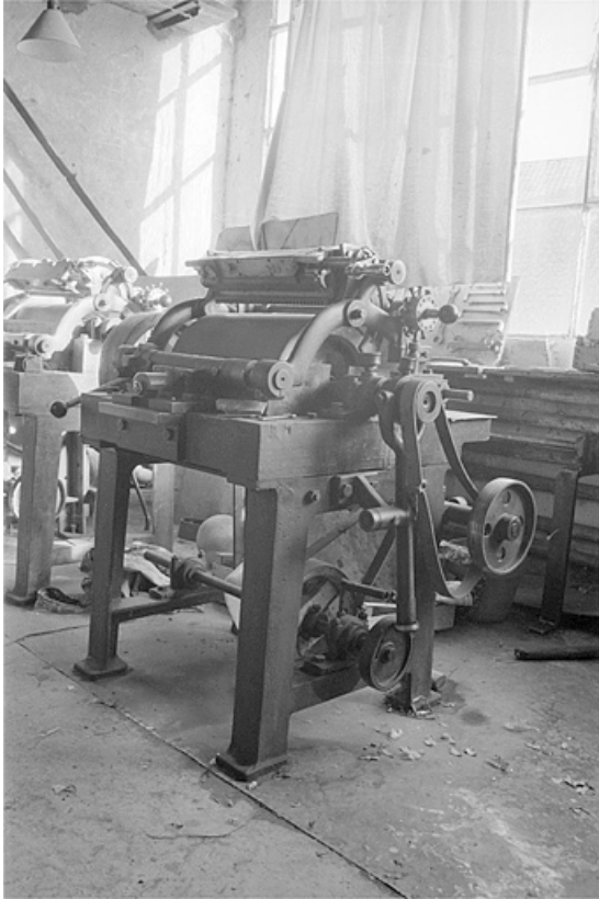
Appareil à cylindre. Porte-pierres baissé.
