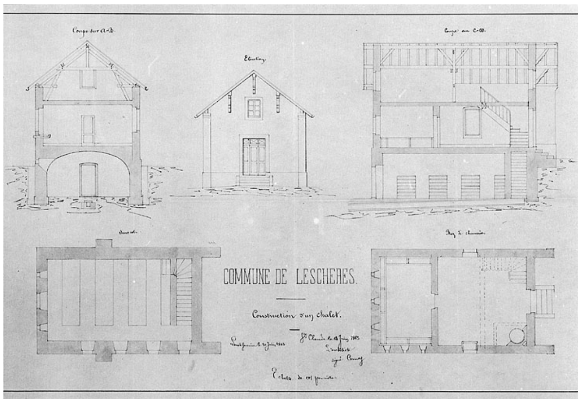
Commune de Leschères, construction d'un chalet [plans, coupes et élévation].
