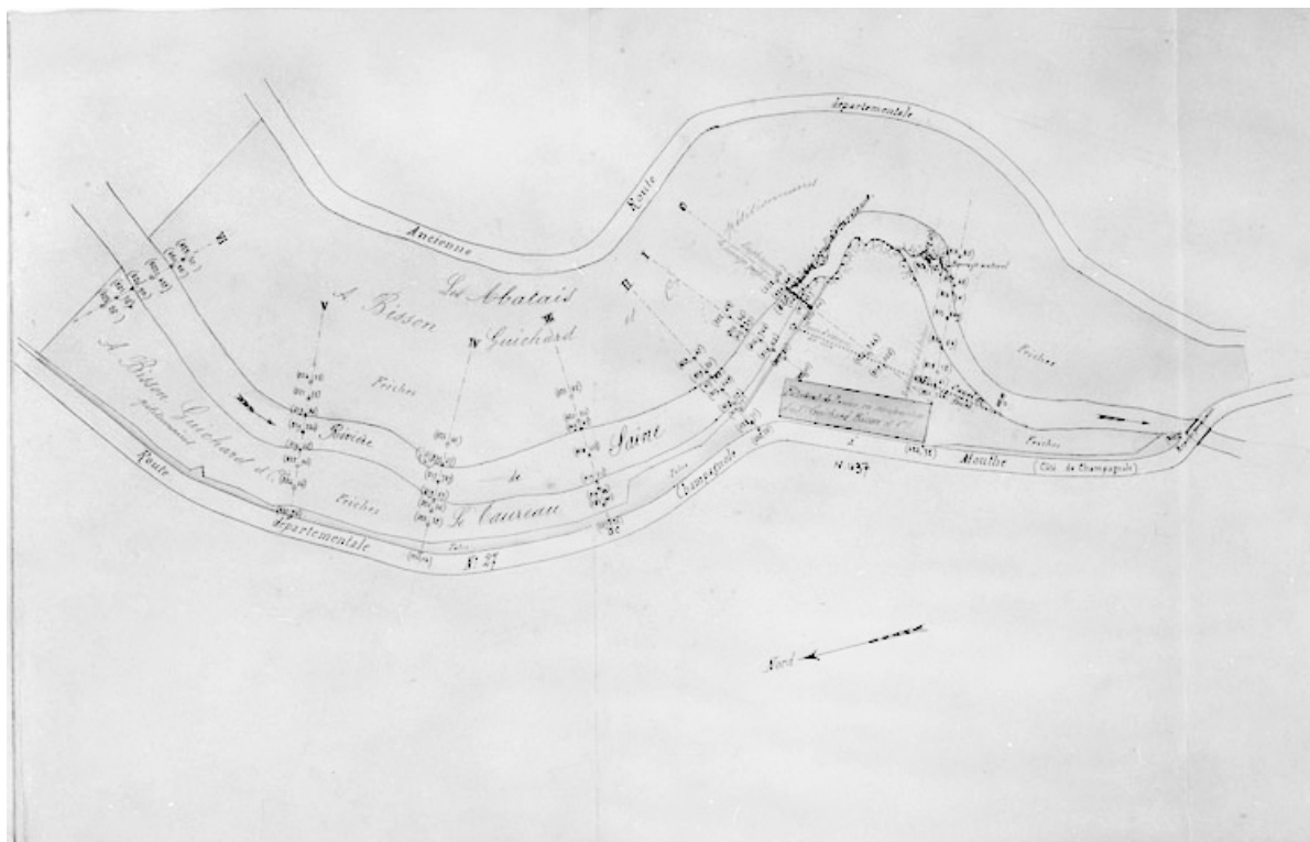
Règlement d'eau de l'usine des sieurs Guichard et Bisson - Plan des lieux.
