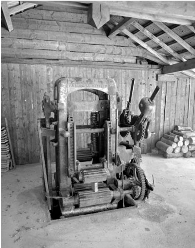
Scie à lames multiples vue de face (les lames ont disparu).
