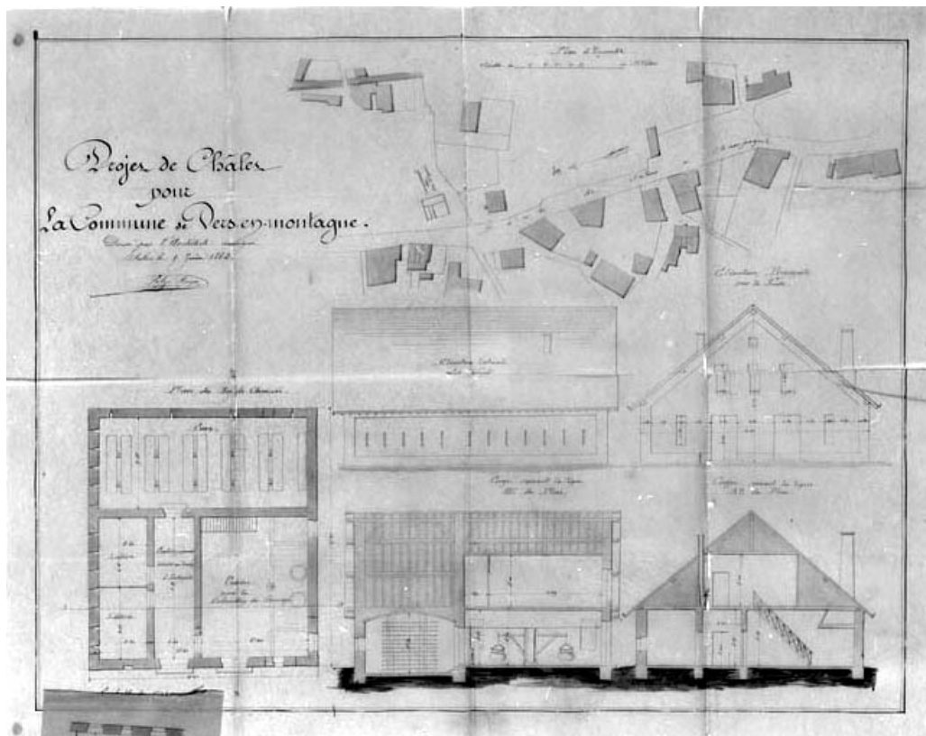
Projet de chalet pour la commune de Vers-en-Montagne [...].
