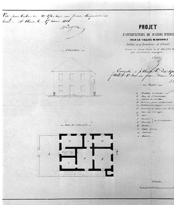
Projet d'appropriation de Maison d'Ecole [...] [plan au rez-de-chaussée et élévation].
