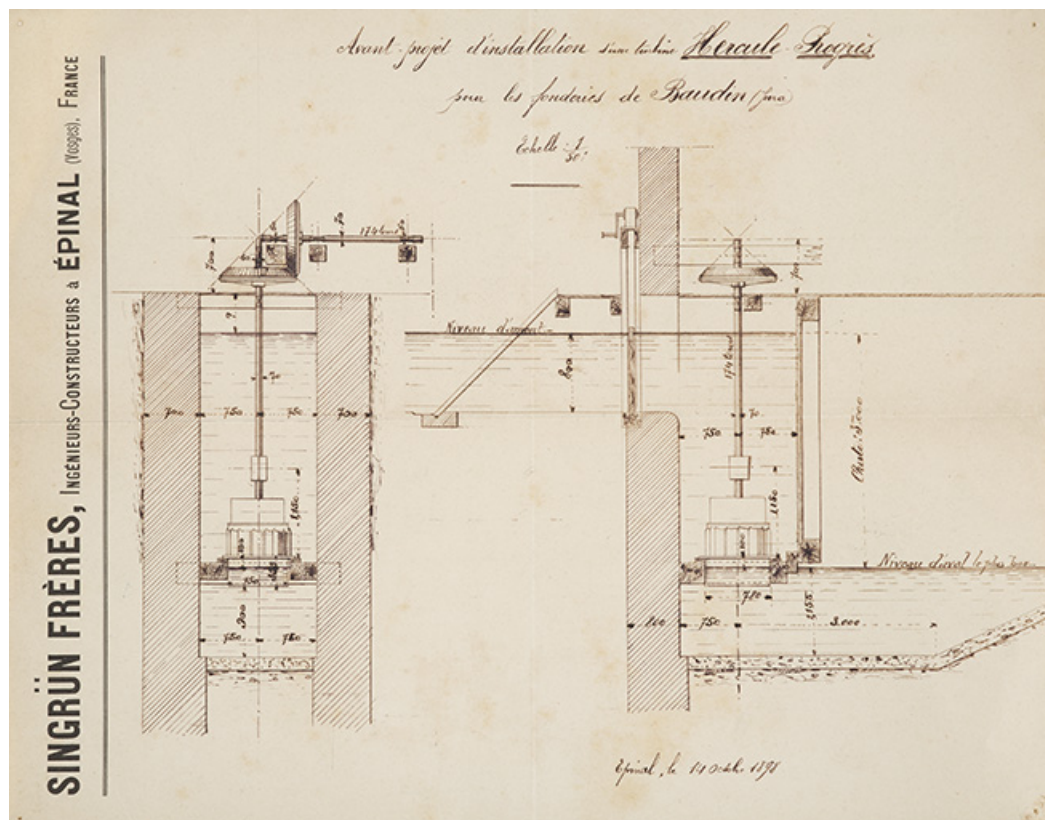
Avant-projet d'installation d'une turbine Hercules-Progress, Epinal, le 14 octobre 1898.
