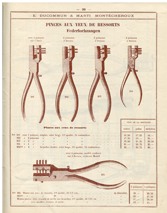
Tarif-album [...] E. Ducommun & Marti successeurs [catalogue de production, p. 39 : pinces pour horloger], [années 1920-1930]. 25, Montécheroux, 1-3 rue de la Planchette
