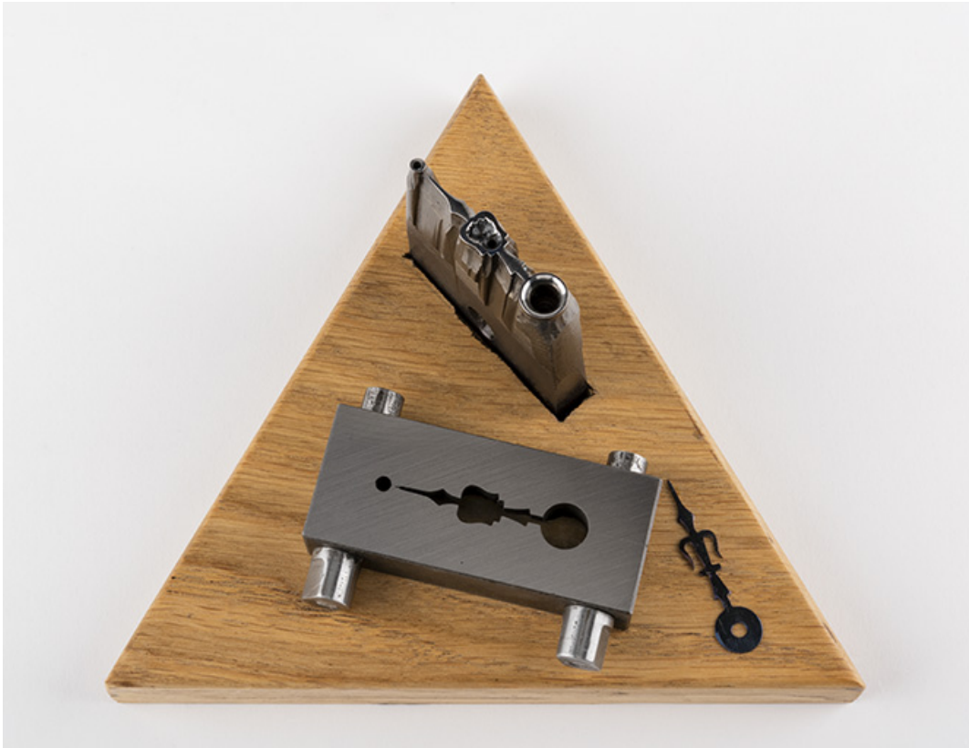
Outils pour découper les aiguilles (collection musée de l'Horlogerie, Morteau). 25, Morteau, 12 rue de la Fraiche
