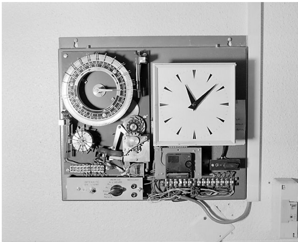
Horloge mère : modules sonnerie et garde-temps.
