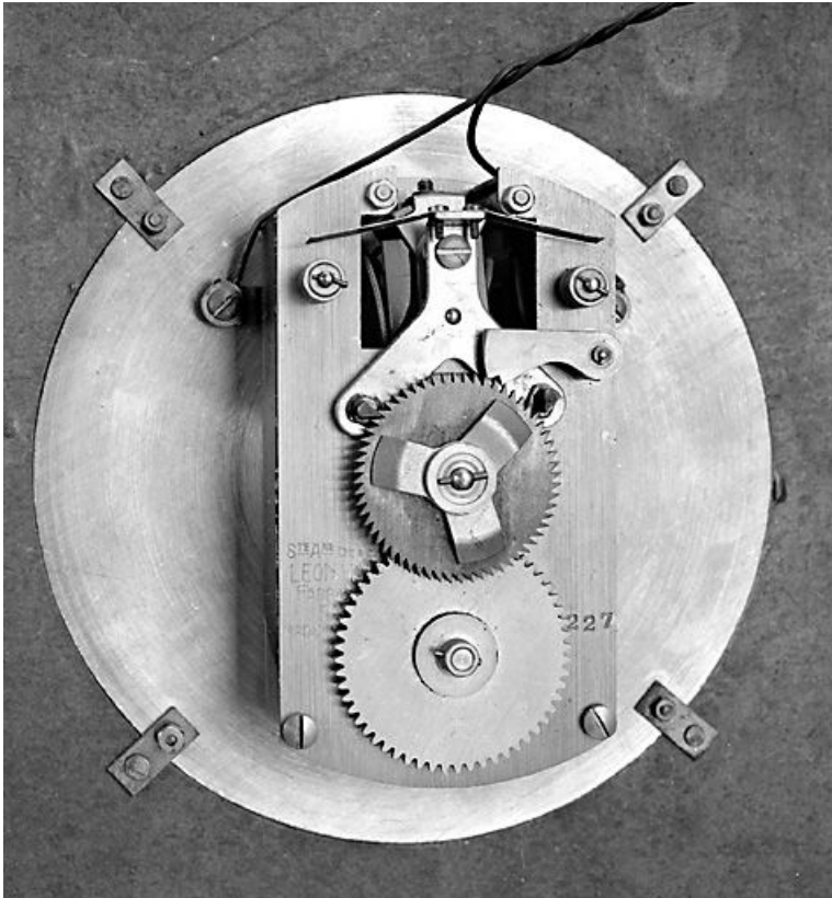
Horloge secondaire : système moteur.
