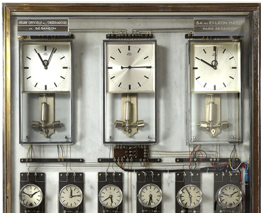
Horloges électriques Hatot, 1934. (Collection musée du Temps, Besançon).
