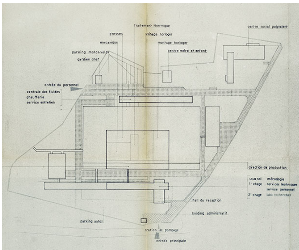
Plan-masse de l'usine, 1957. 25, Besançon chemin de Palente
