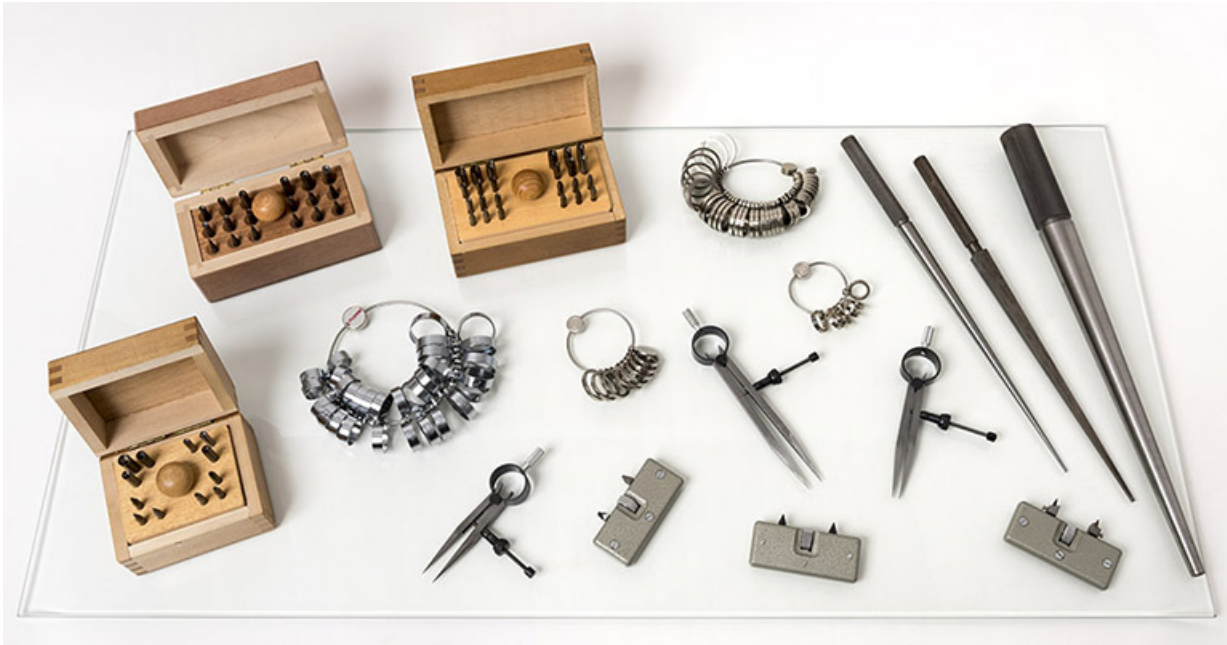
Production de la société Grandidier : jeux de fraises, triboulets, baguiers, compas et clés à ouvrir les fonds de boîte de montre. 25, Grand'Combe-Château, 14 rue les Grands Saules, lieudit : les Forges
