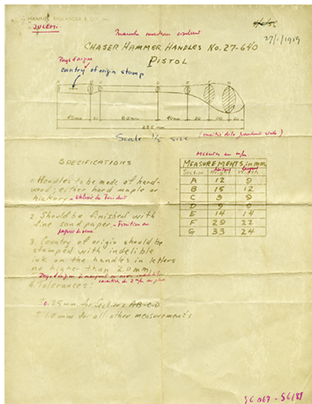
Dessin technique d'un manche de marteau de ciseleur envoyé par la société Hammel, Riglander & Co, 27 janvier 1959. 25, Les Gras, 12-14 rue les Jean-Jacquot, lieudit : les Jean-Jacquot
