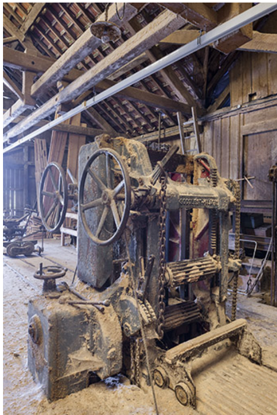
Châssis multilames vu de trois quarts arrière.
