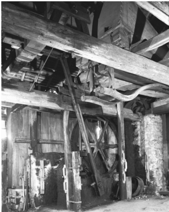
Vue rapprochée des mécanismes et des soufflets de trois quarts gauche.
