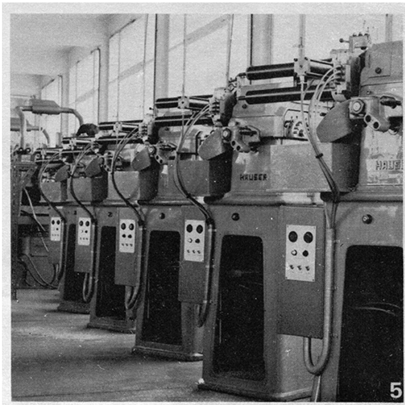
[France Ebauches] Batterie de machines à contourner automatiques, 1970.
