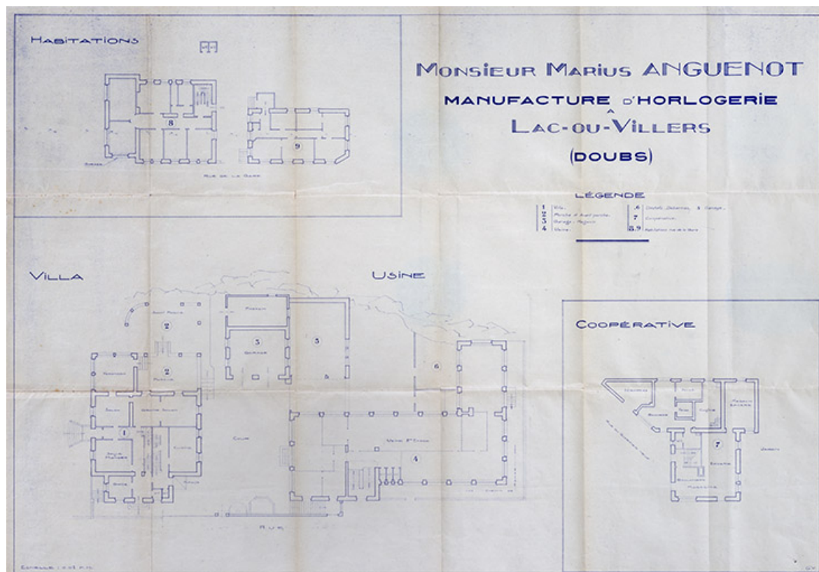
Monsieur Marius Anguenot. Manufacture d'horlogerie à Lac-ou-Villers (Doubs) [plans de la villa et l'usine rue de la Perrière, des habitations rue de la Gare et d'une coopérative rue du Quartier neuf], 2e quart 20e siècle.
