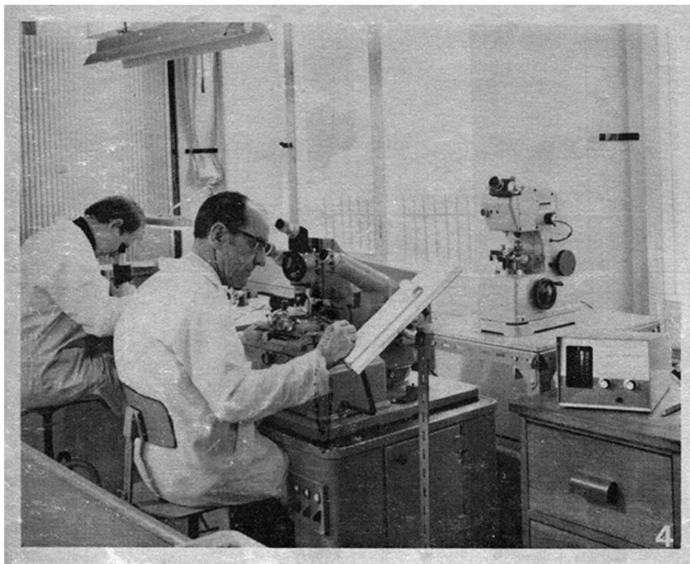
[France Ebauches] Atelier de contrôle, usine n° 4, 1970.
