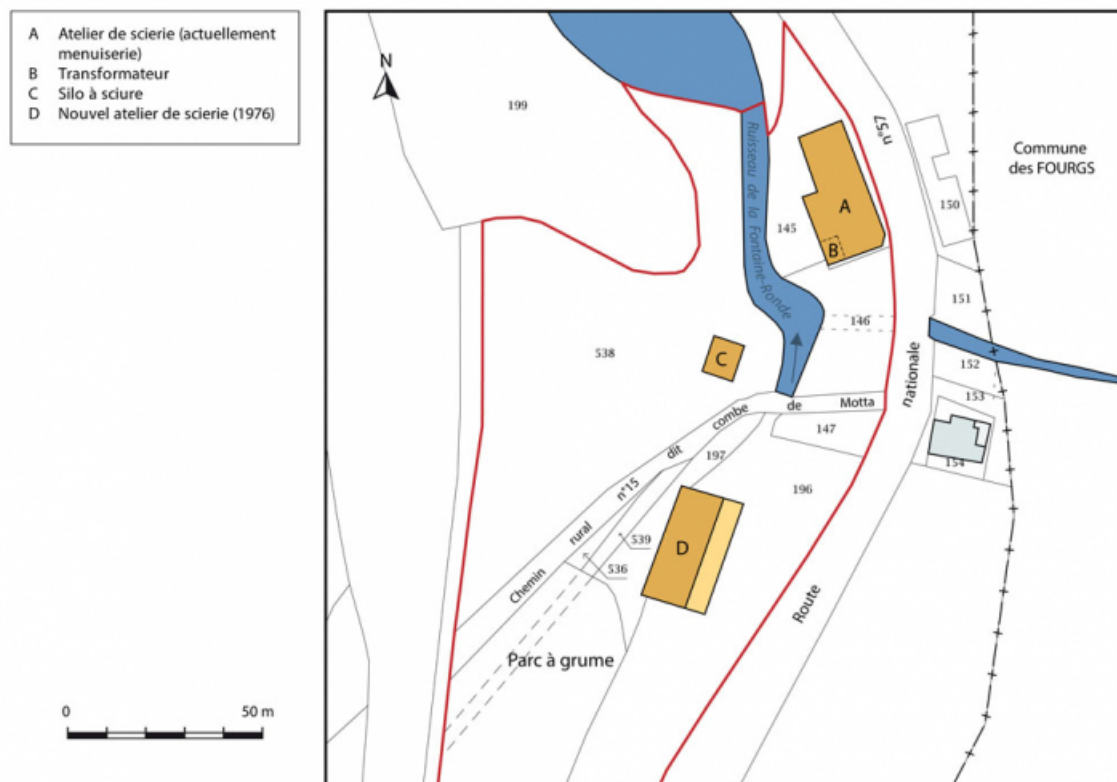
Plan-masse et de situation. Extrait du plan cadastral, 2015, section D. 25, La Cluse-et-Mijoux, lieudit : la Gauffre
