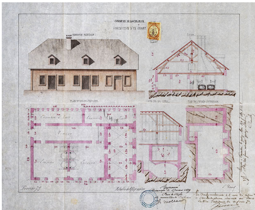
Construction d'un chalet [plans, coupes, élévation], 1879.
