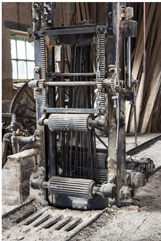
Châssis de scie. Partie basse.
