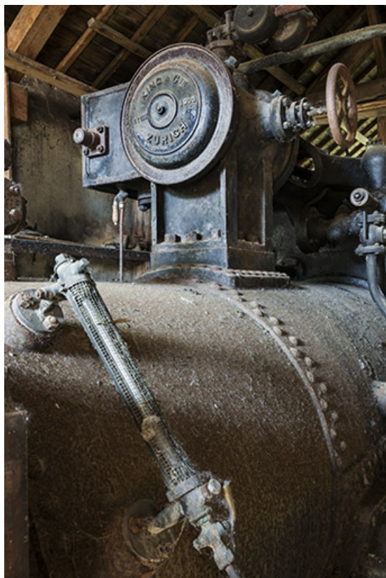
Détail du cylindre.
