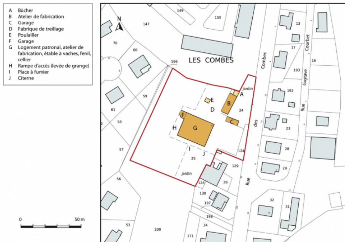
Plan-masse et de situation. Extrait du plan cadastral, 2015, section AD. 25, Maîche, 6 et 8 rue des Combes
