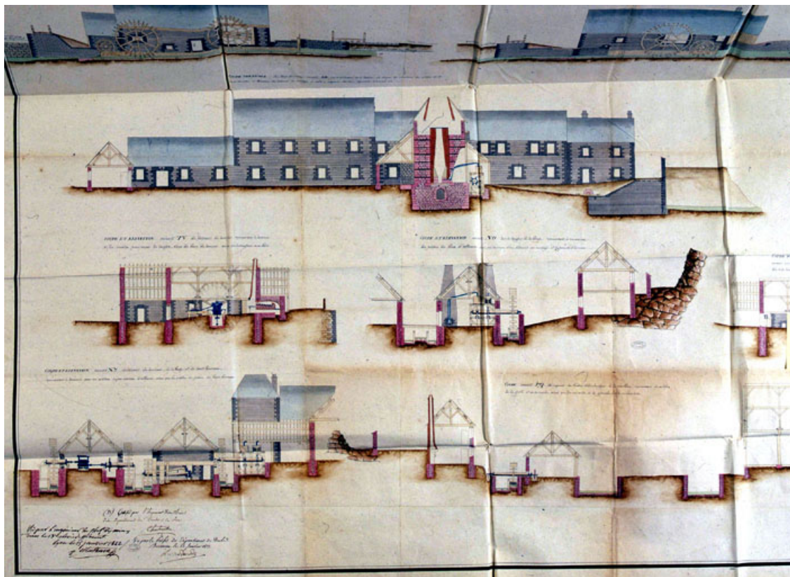
Coupe en long de l'atelier des laminoirs en 1821.
