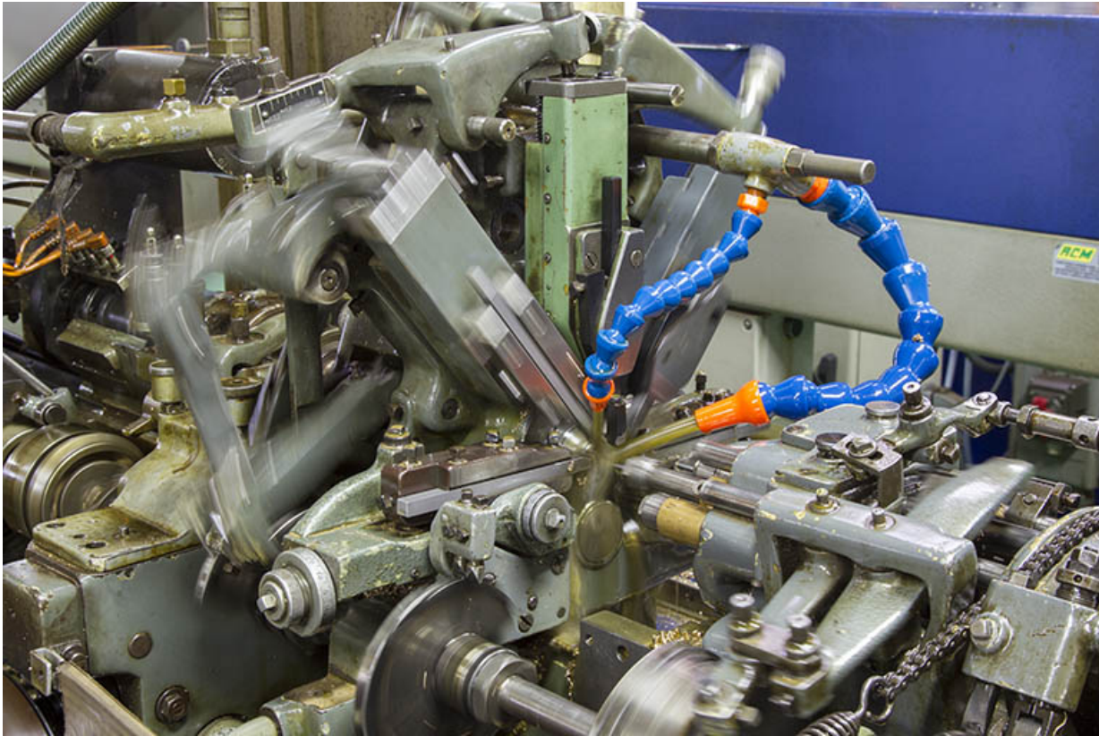
Machine à décolleter ancienne en fonctionnement.
