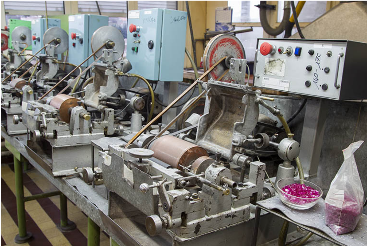
Atelier de taille du rubis : machines à usiner par abrasion (machines suisses Bocadero). 25, Charquemont, 18 rue de Besançon
