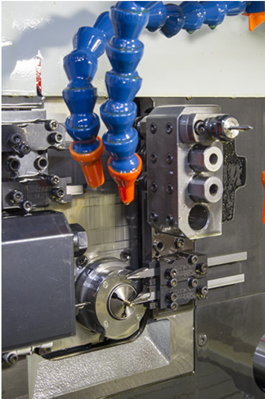
Machine à décolleter récente : installation de lubrification de la pièce et des outils.
