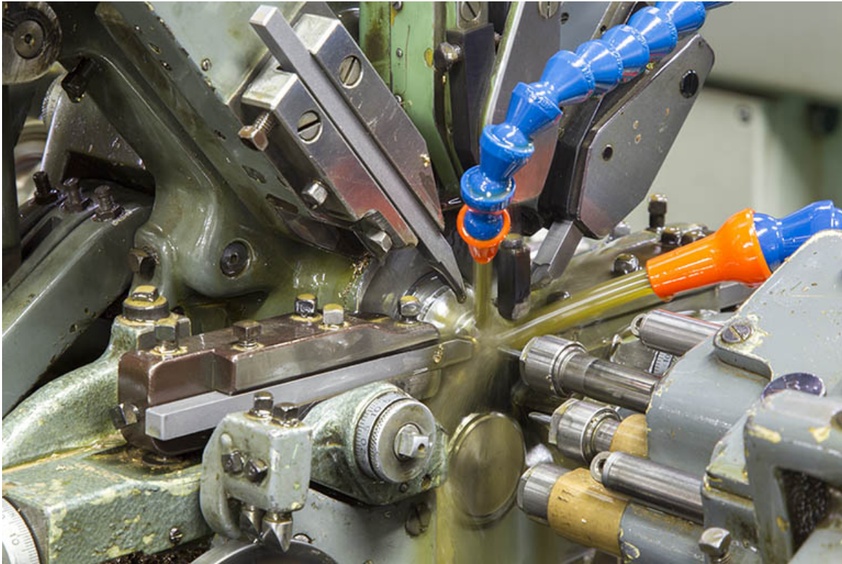
Machine à décolleter ancienne : lubrification de la pièce et des outils.
