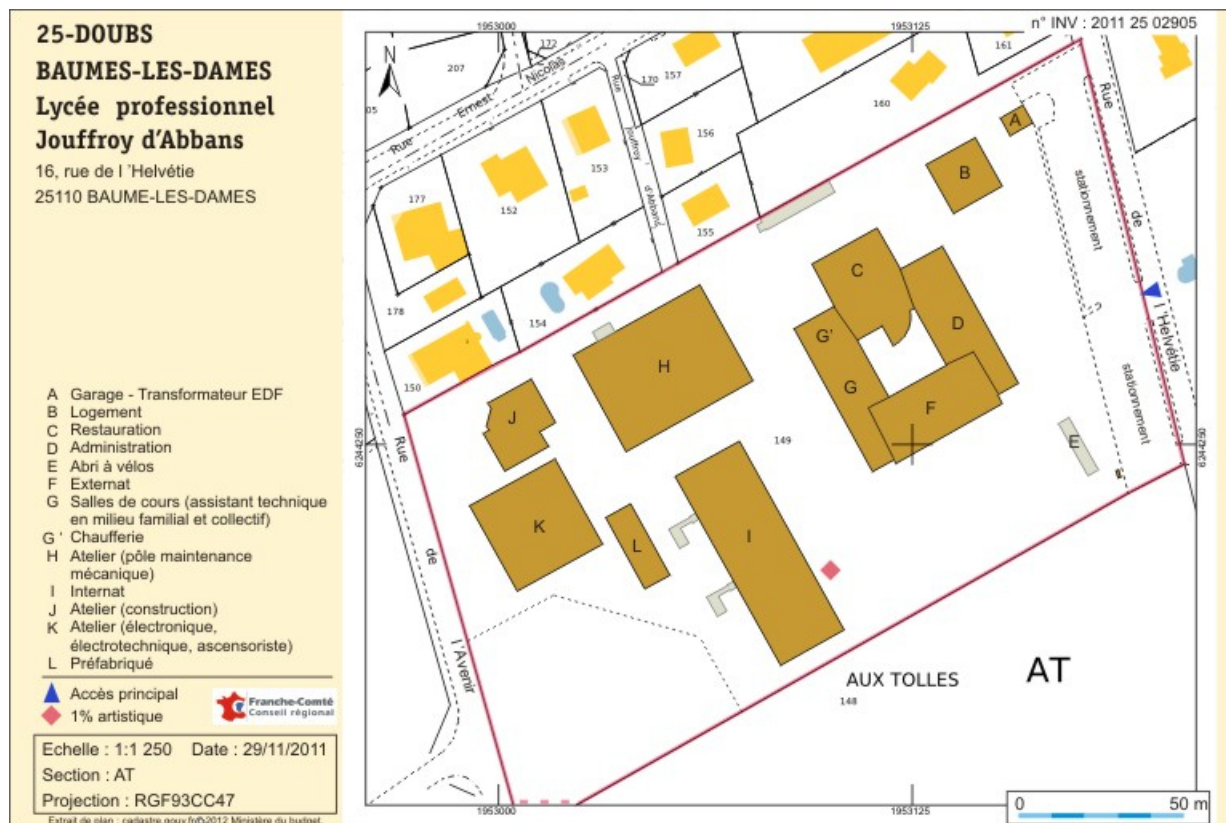
Plan-masse et de situation. Extrait du plan cadastral numérisé, section AT, échelle 1:1250. 25, Baume-les-Dames, 16 rue de l' Helvétie
