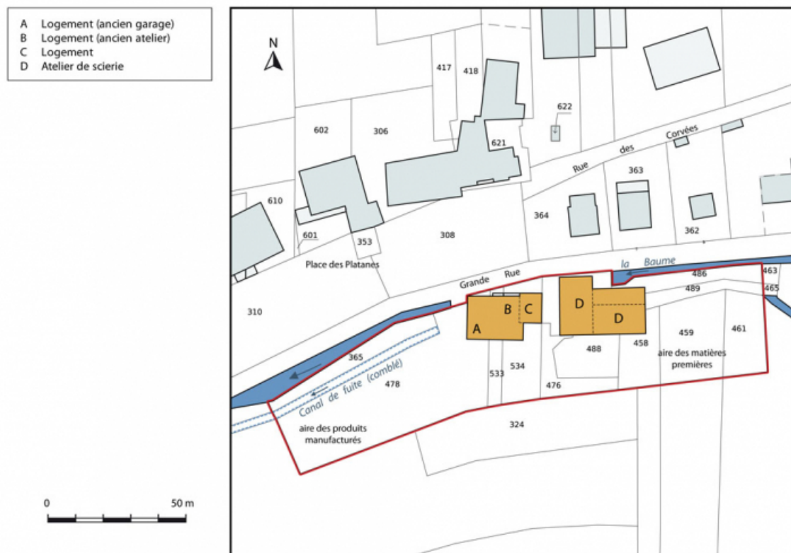
Plan-masse et de situation. Extrait du plan cadastral, 2015, section B. 25, Sancey-le-Long, 2 Grande-rue
