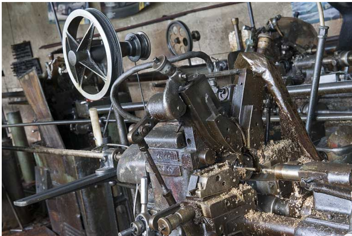
Atelier primitif. Partie supérieure d'une machine à décolleter.
