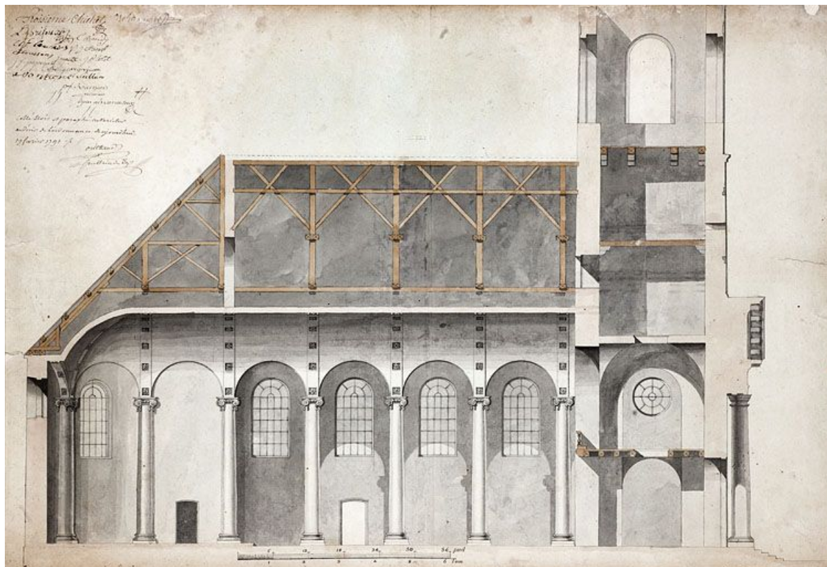
[Coupe longitudinale de l'église]. S.d. [1789].
