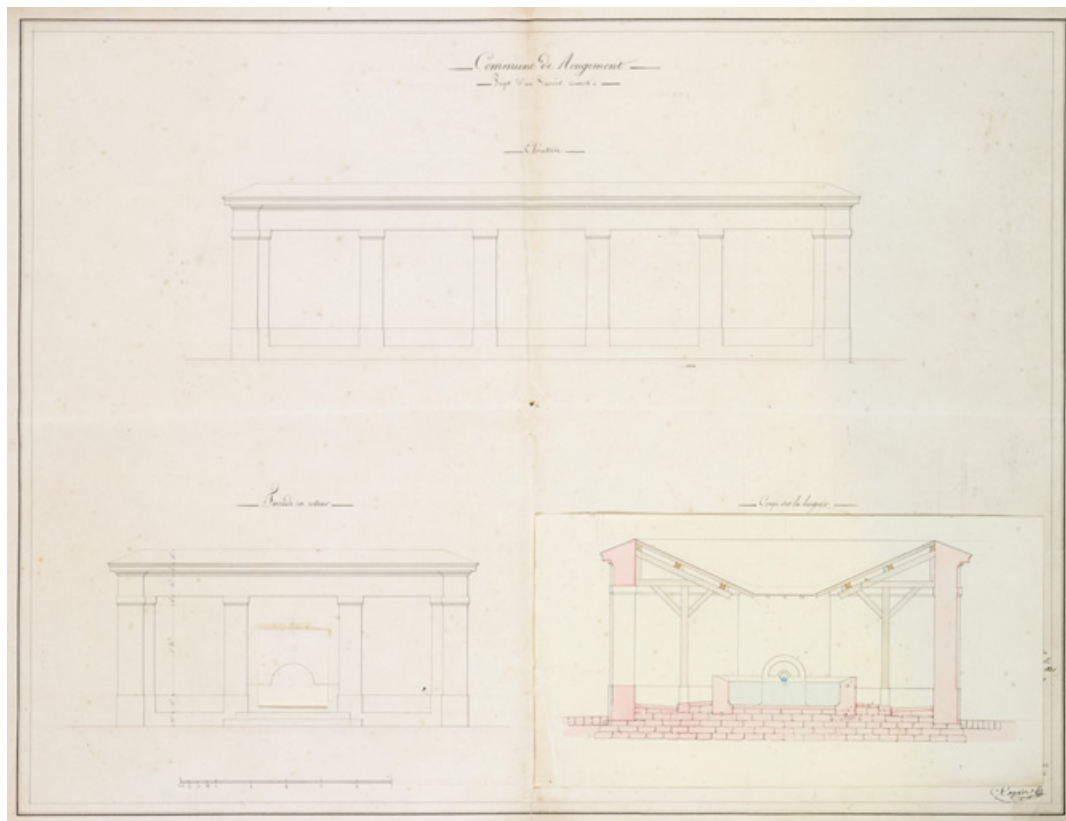
Commune de Rougemont. Projet d'un lavoir couvert. Façade en retour. Coupe sur la largeur. 1831. 25, Rougemont rue du Lavoir
