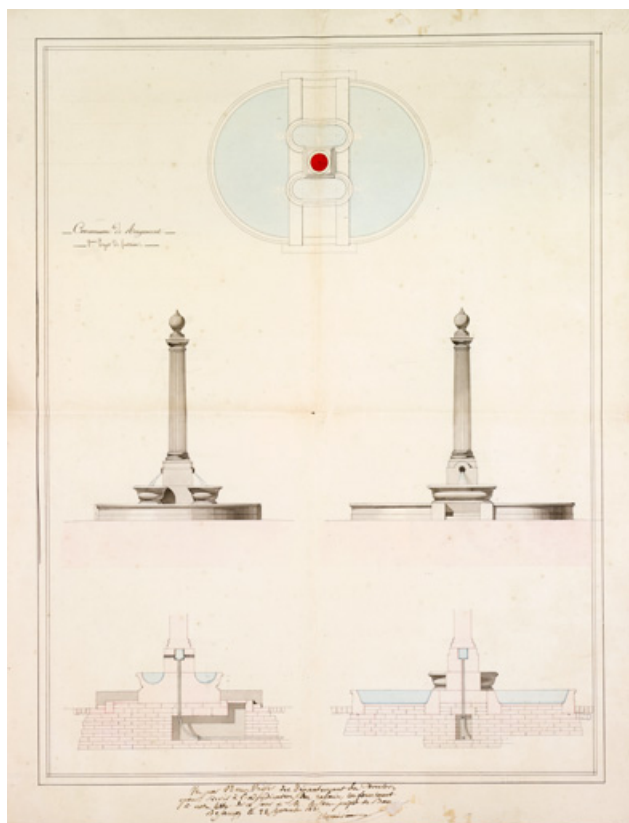
Commune de Rougemont. 2e projet de fontaine. 1831.
