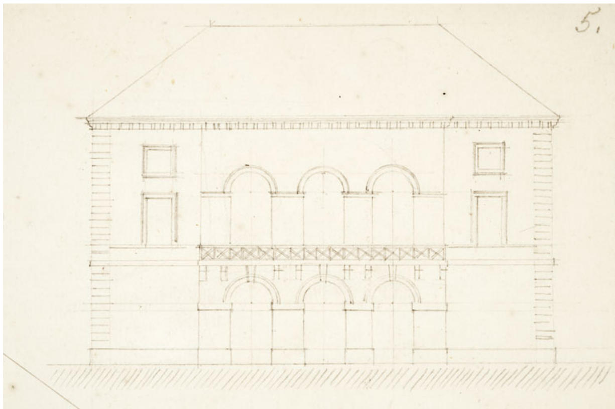
Croquis du projet de la façade latérale, côté lavoir.
