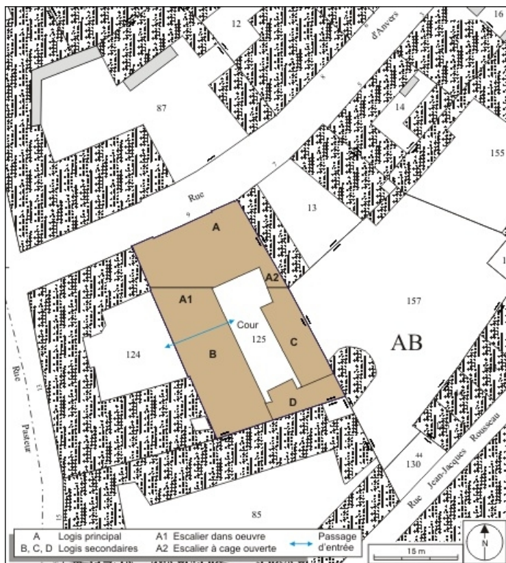
Plan masse et de situation. Extrait du plan cadastral, 1974, section AB. 25, Besançon, 9 rue d' Anvers, lieudit : îlot d' Emskerque
