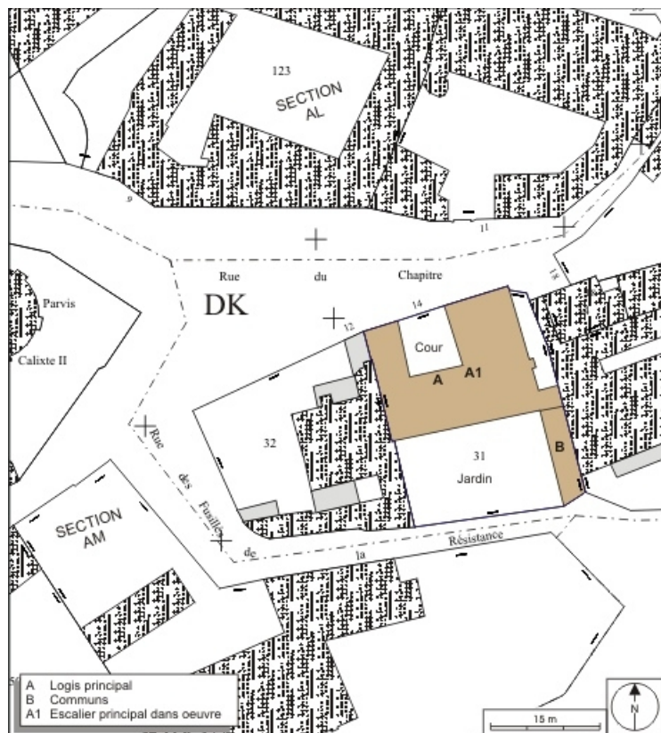
Plan masse et de situation. Extrait du plan cadastral, 1974, section AL. 25, Besançon, 14 rue de la Convention, lieudit : îlot Boitouset
