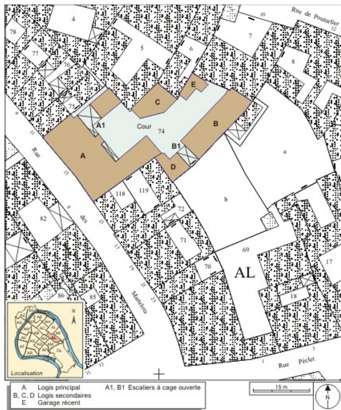
Plan masse et de situation. Extrait du plan cadastral, 1974, section AL. 25, Besançon, 13 rue des Martelots, lieudit : îlot des Martelots
