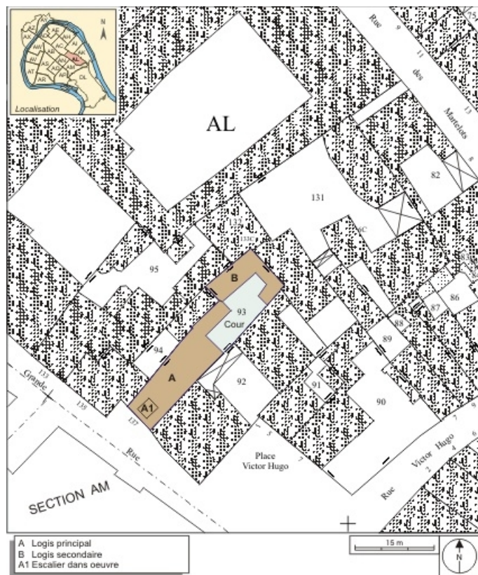
Plan masse et de situation. Extrait du plan cadastral, 1974, section AL. 25, Besançon, 137 Grande Rue, lieudit : îlot Saint-Maurice
